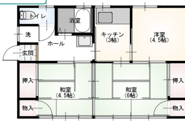
間取り図
