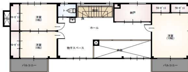
3階 平面図 S:1/100
